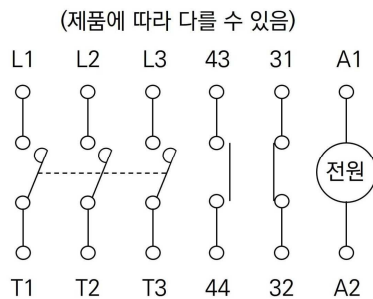
[MC 내부결선도]
