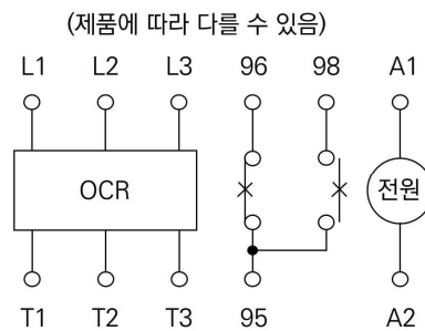
[OCR 내부결선도]
